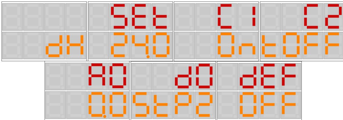
Interfaccia utente EPJ LCD e EVJ LCD
