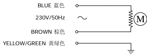
Wiring diagram 接线图
