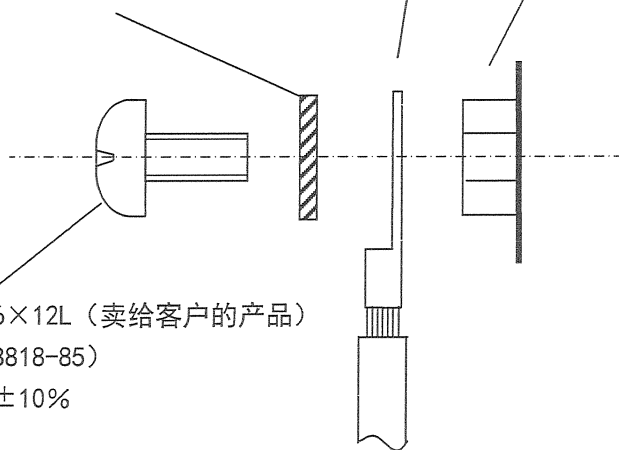
接地端子安装详细图
